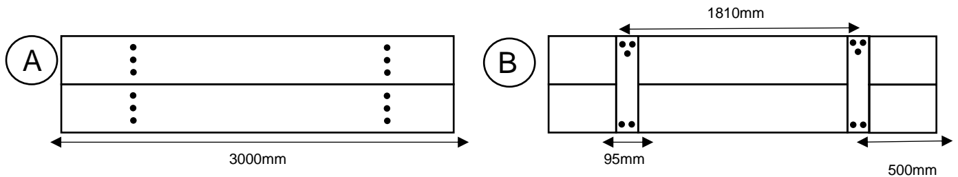
Piirroskuvassa 2 A: on kuvattu edestäpäin kaukalon laidan 3 metriä pitkä osa ja kuvassa 2 B näkyy samainen osa takaa päin kuvattuna. Kuvasta näkyy samalla 2 tukipuurakennetta.
