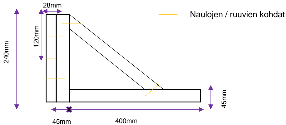
Piirroskuva 1: Kuvassa on havainnollistettu sivulta päin kuinka laudat ja niiden tukipuut kiinnitetään toisiinsa.
